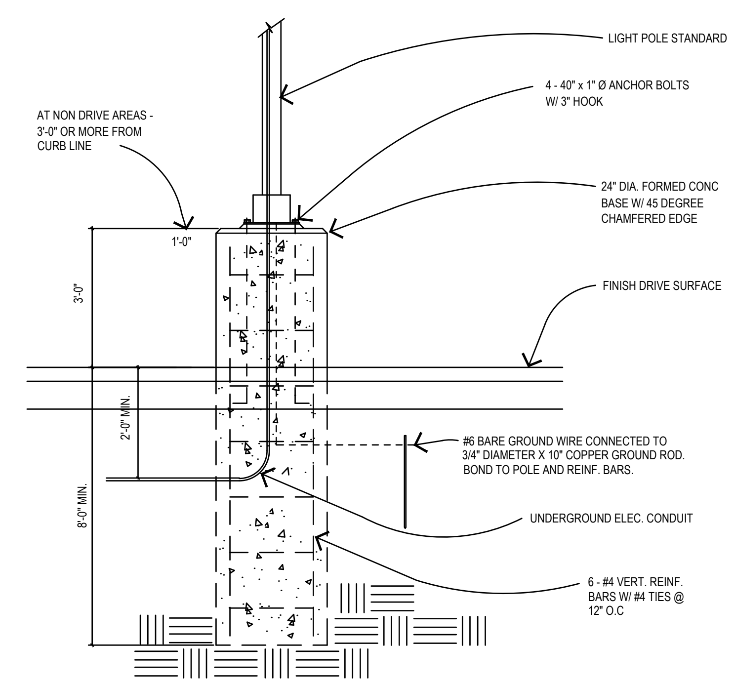
1 TALL POLE BASE DP-1 SCALE: NONE
