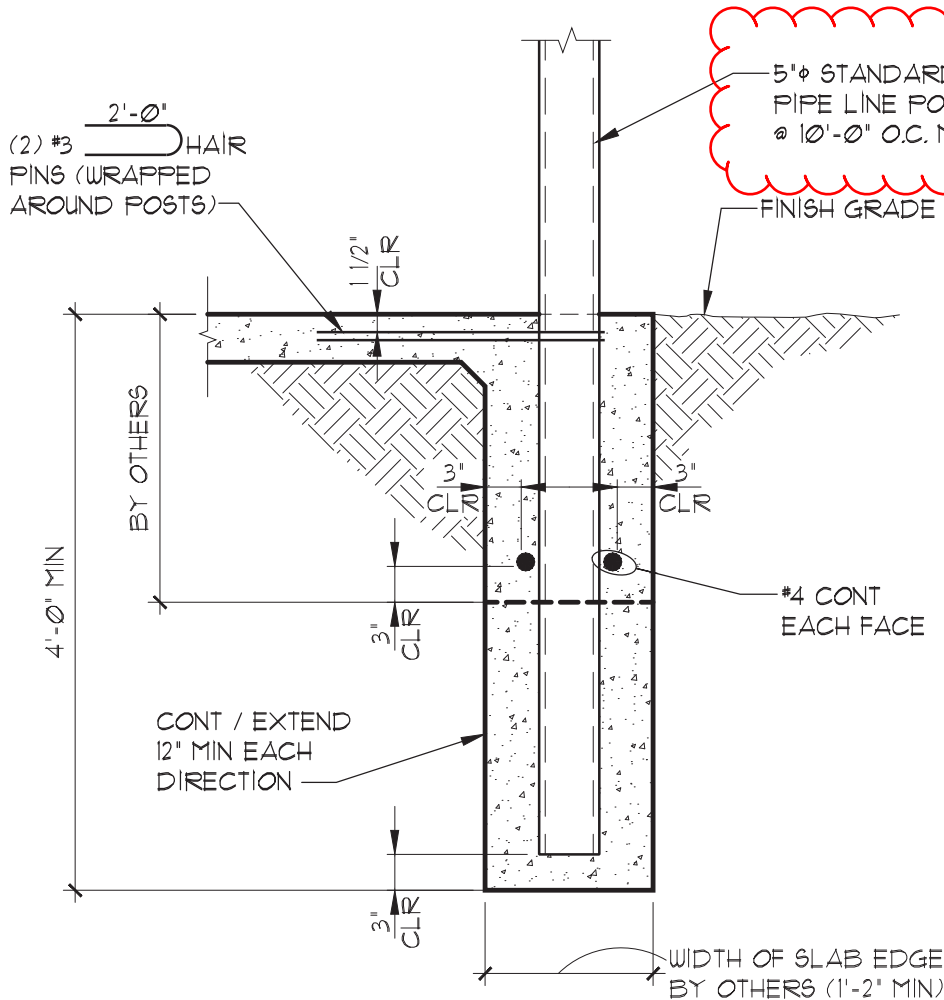
A DETAIL SCALE: 3/4" = 1'-0"
