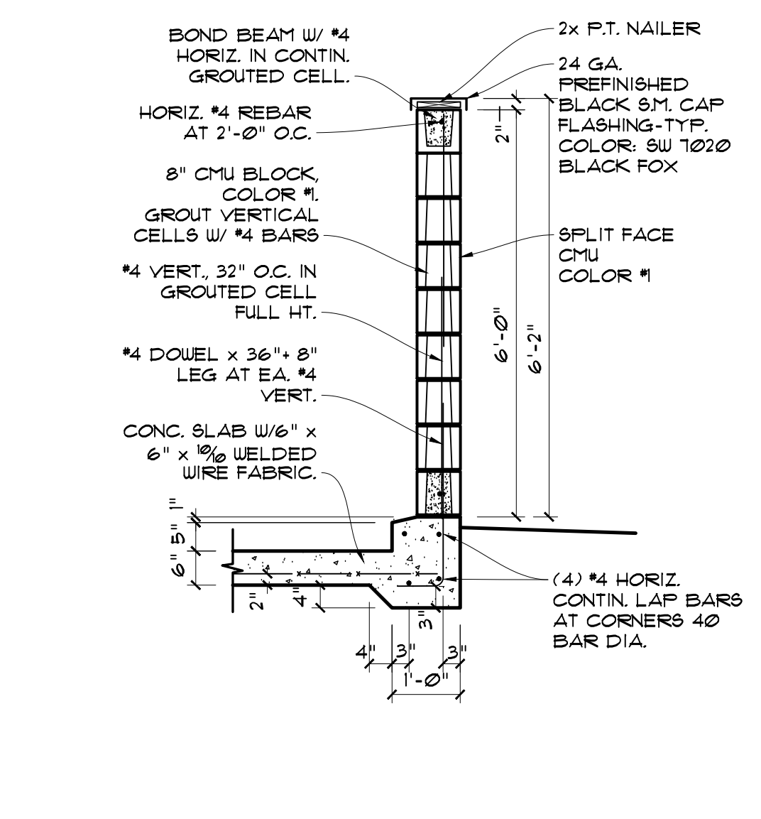
7 DETAIL - WALL A100 SCALE: 1/2" - 1'-0"
