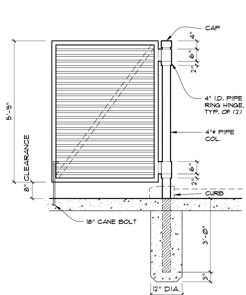
8 DETAIL - GATE A100 SCALE: 1/2" - 1'-0"
