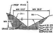
SWALE SECTION A-A TYPICAL DETAIL SCALE: N.T.S.
