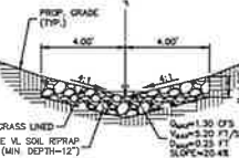
POND MINOR SWALE TYPICAL DETAIL SCALE: N.T.S.
