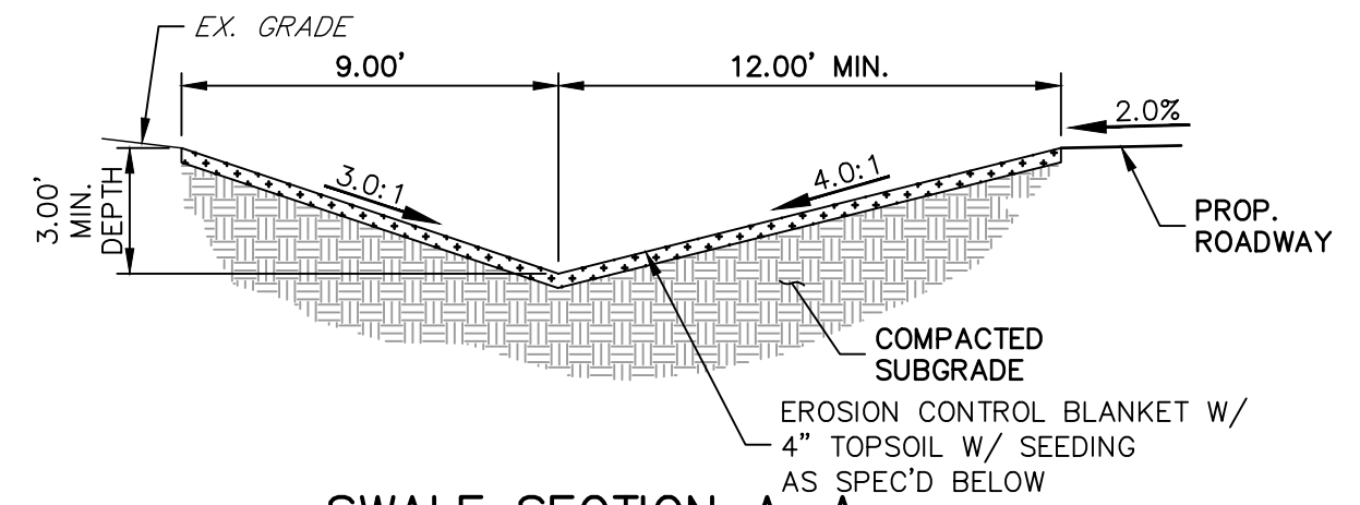
SWALE SECTION A-A SCALE: 1" = 5'
