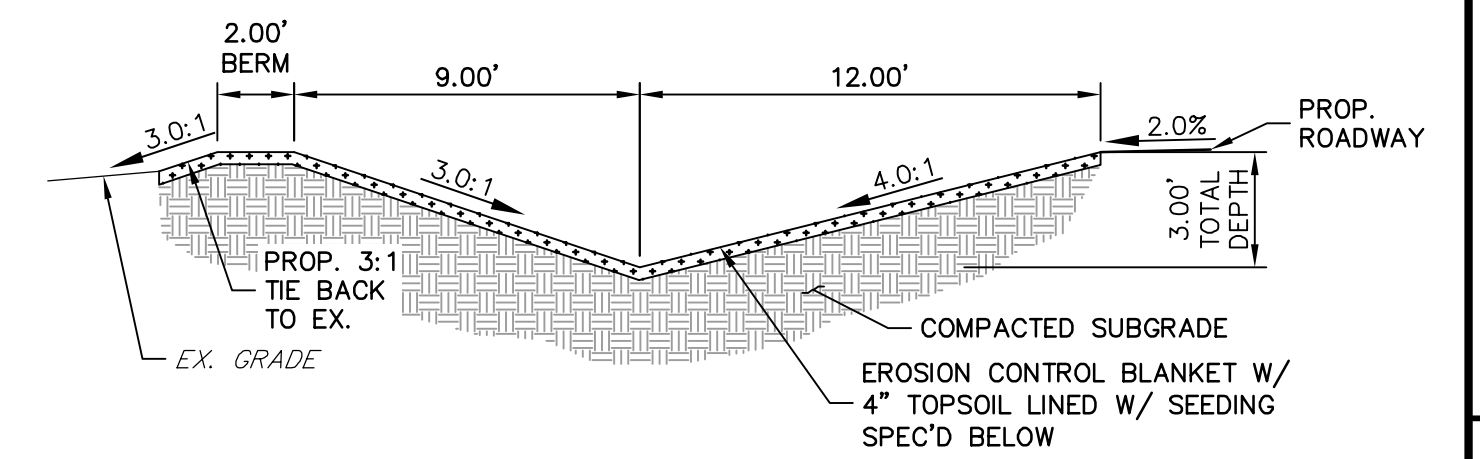
SWALE SECTION B-B SCALE: 1" = 5'
