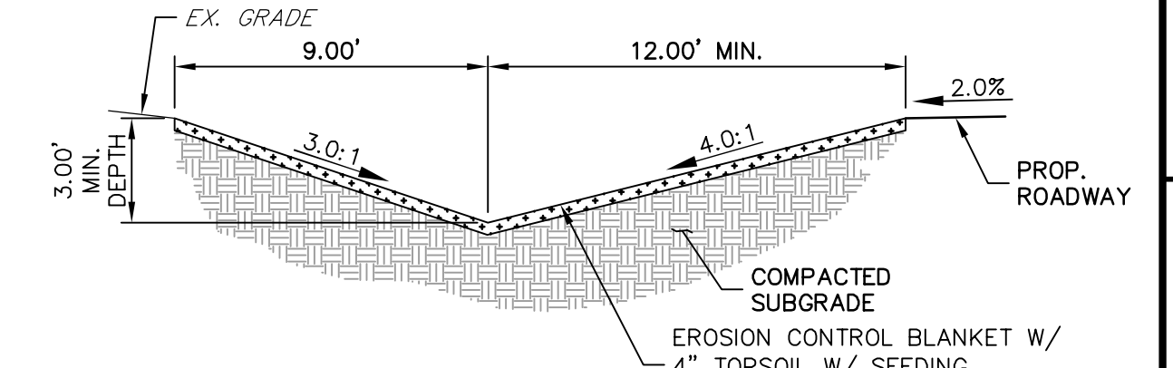
SWALE SECTION A-A SCALE: 1" = 5'
