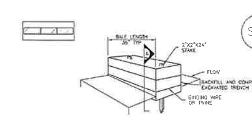
SBB-1. STRAW BALE
