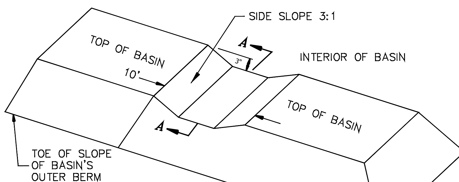
SPILLWAY CROSS SECTION SECTION N.T.S.
