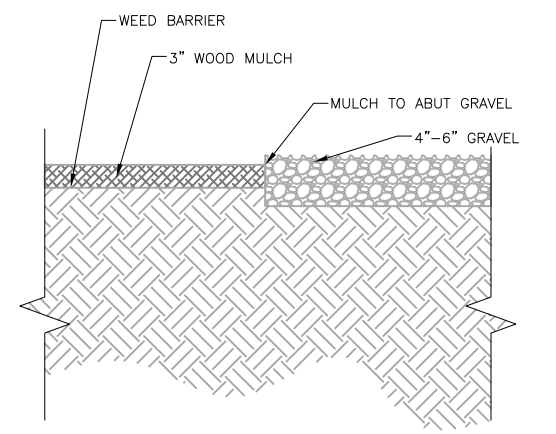
E GRAVEL @ MULCH LS2 SCALE: N.T.S.
