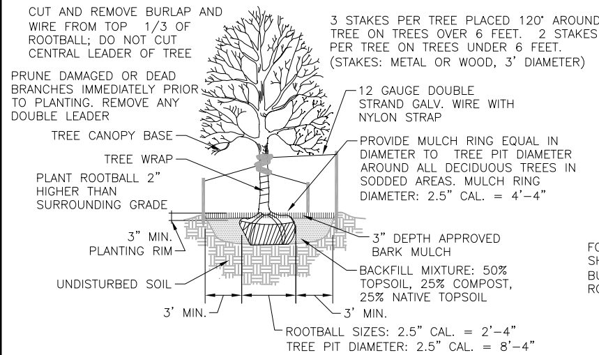
A TREE PLANTING LS2 SCALE: N.T.S.
