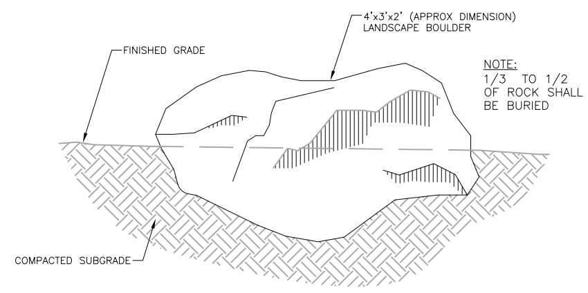
C LANDSCAPE BOULDER LS2 SCALE: N.T.S.
