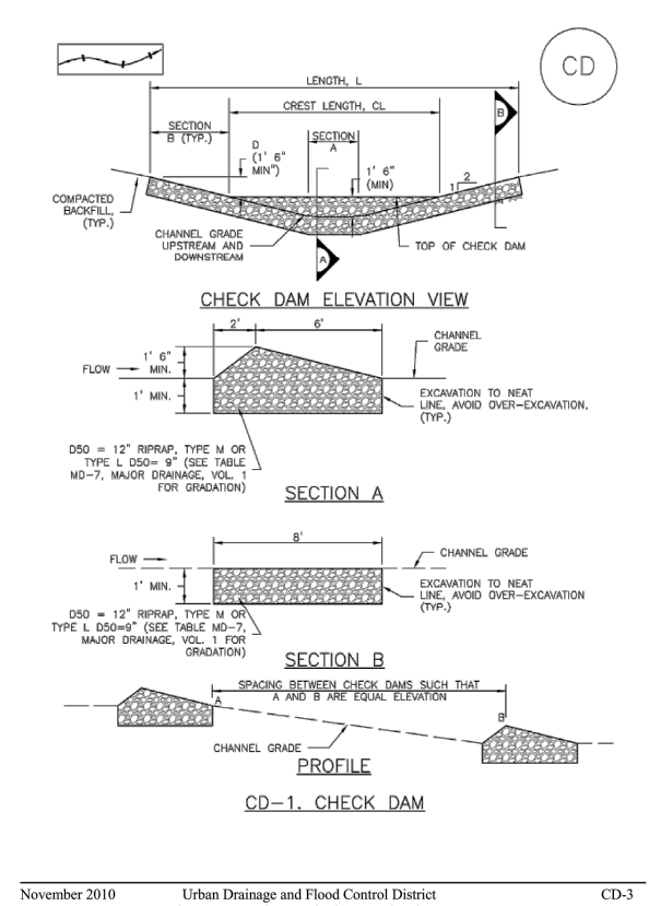
EC-12 Check Dams (CD)
