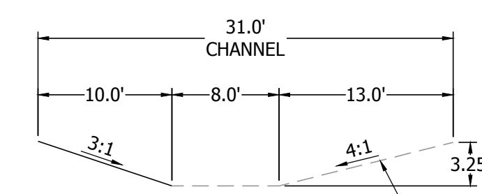
CHANNEL E SECTION A-A SCALE: 1" = 10'
