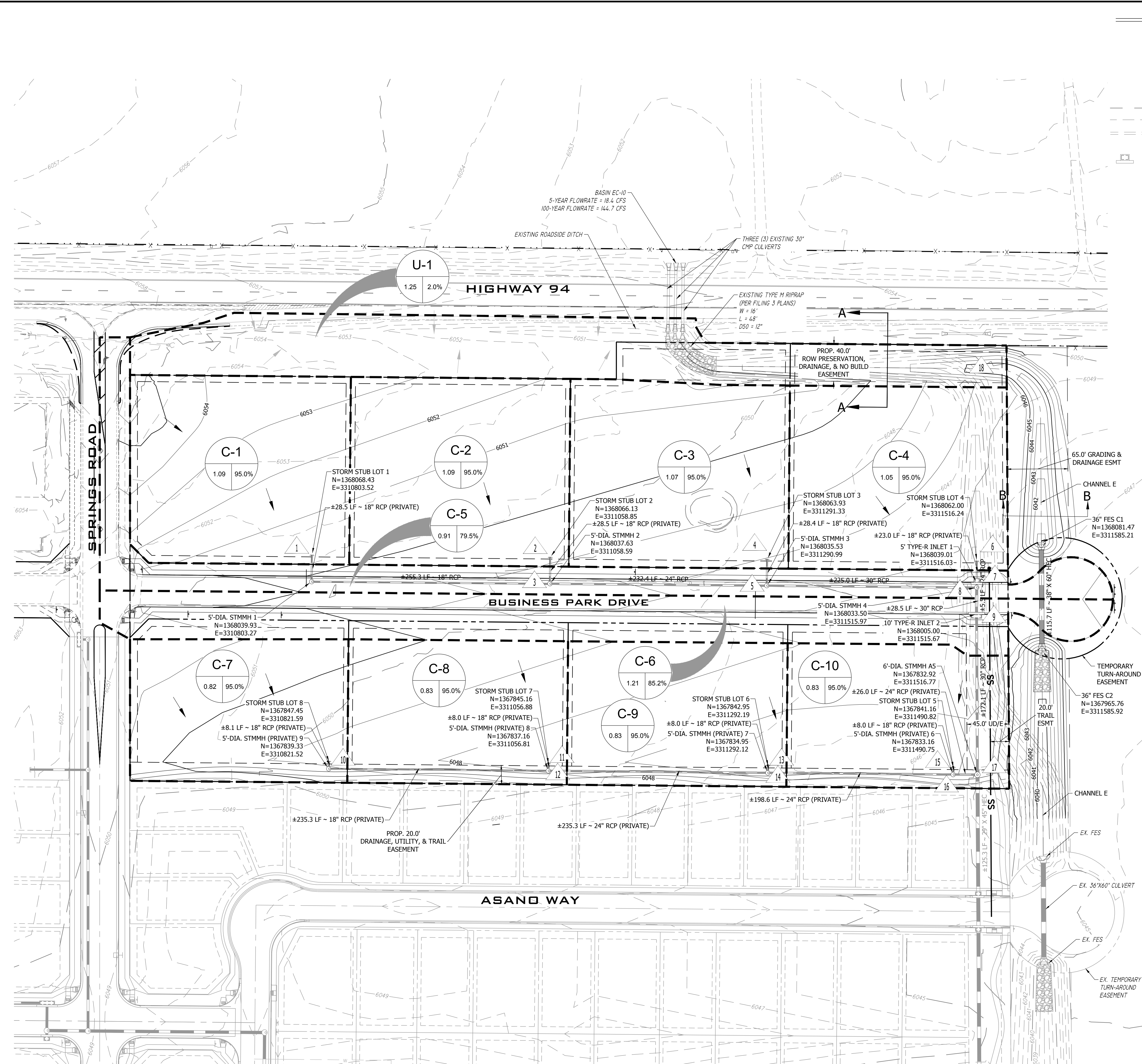
SCALE: 1" = 50'
