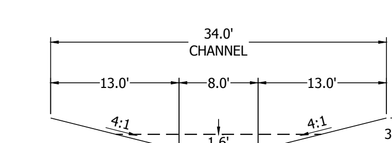
CHANNEL E SECTION B-B SCALE: 1" = 10'
