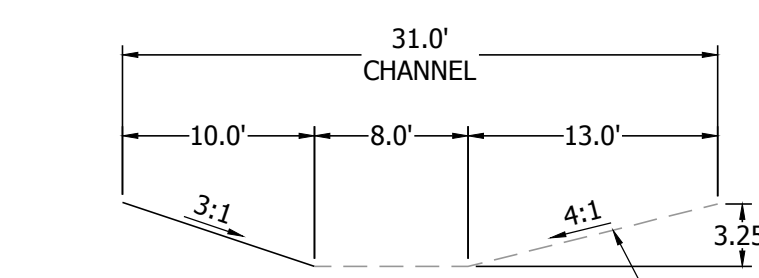
CHANNEL E SECTION A-A SCALE: 1" = 10'
