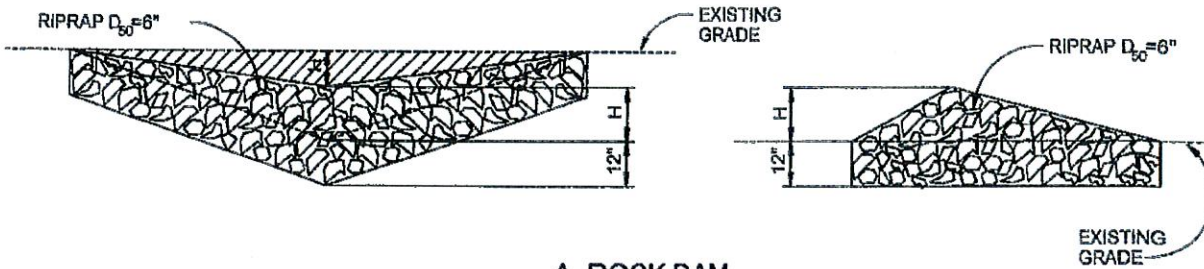
A. ROCK DAM
