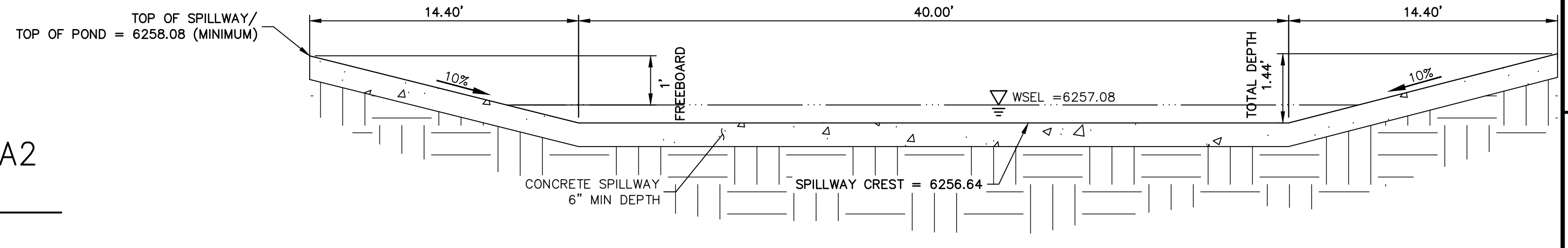
POND A EMERGENCY OVERFLOW SPILLWAY SCALE: N.T.S.
