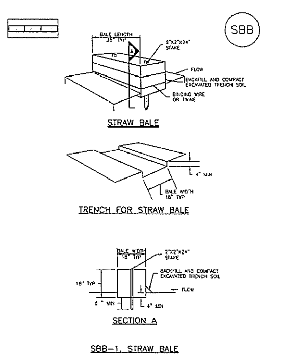
SBB-1. STRAW BALE
